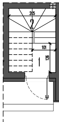
RZUT PARTERU
